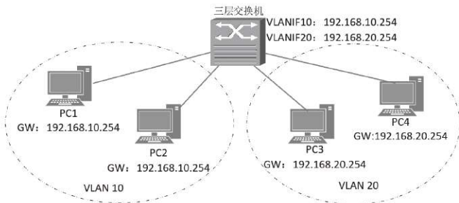
图 4-10 三层交换
