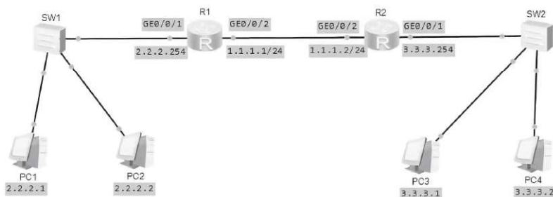
图 4-11 实训拓扑图
