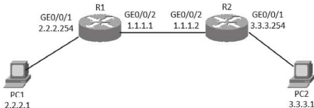
图 4-5 网络拓扑
