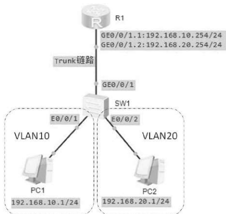
图 4-12 实训拓扑图
