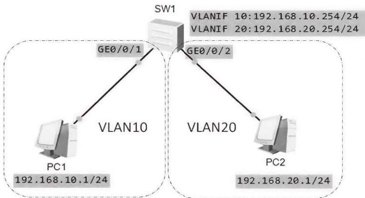
图4-14 实训拓扑图
