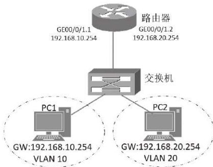
图 4-9 单臂路由
